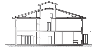
SEZIONE B-B scala 1:100
