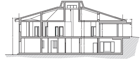
SEZIONE B-B scala 1:100
