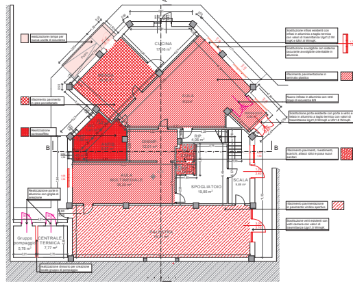
_PIANTA PIANO SOTTOSTRADA scala 1:100
