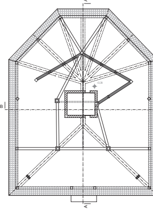
_PIANTA SOTTOTETTO scala 1:100
