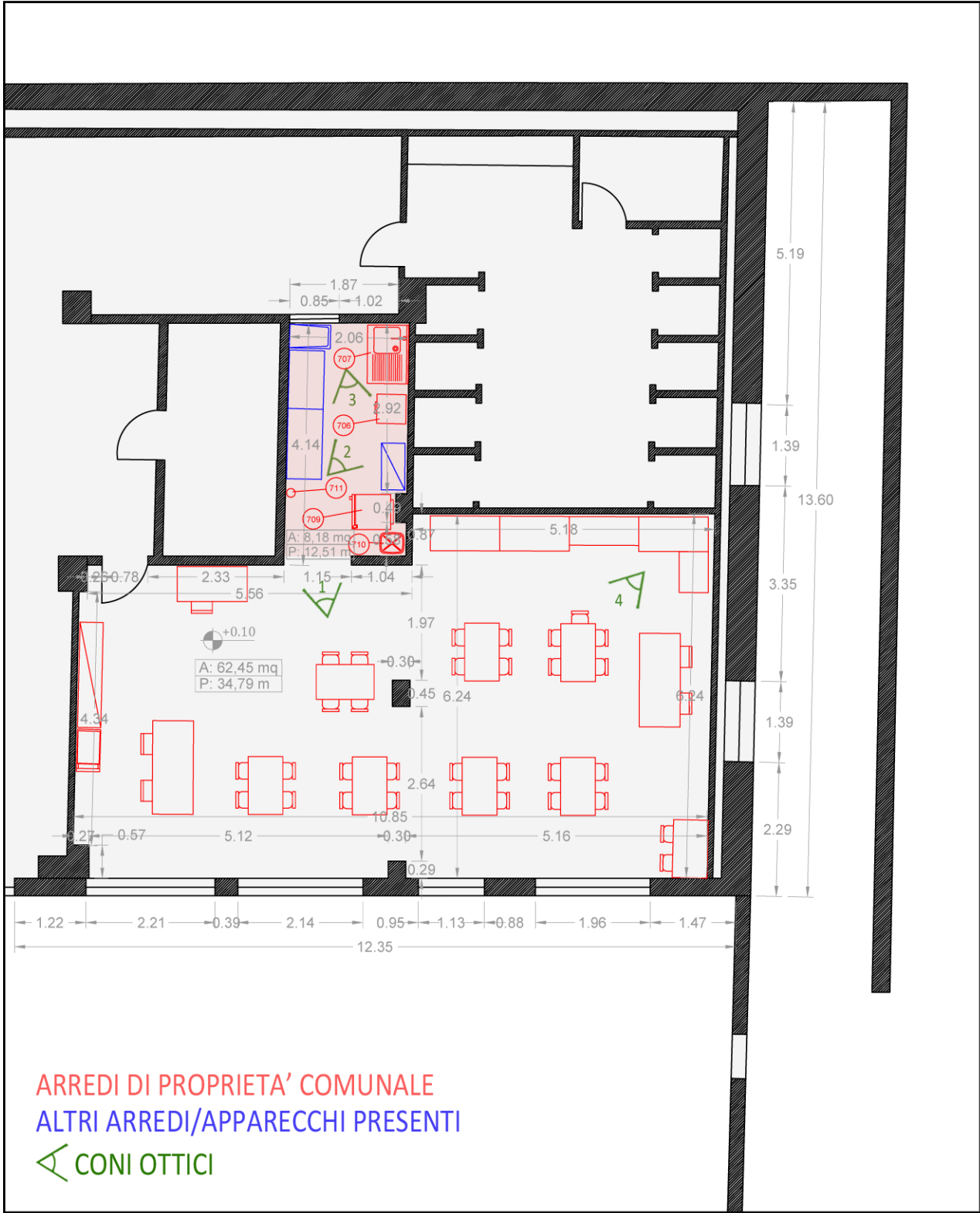
PLANIMETRIA LOCALI MENSA SCALA 1:100
